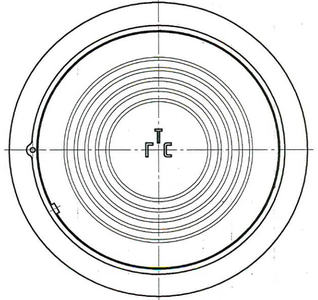
Люк телефонный тип Т ГОСТ 8591-76
